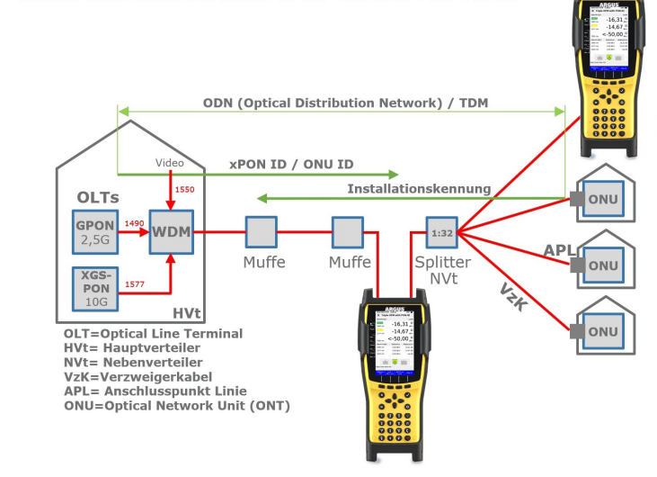
Aufbau eines koexistierenden GPON- und XGS-PON-Netzes
