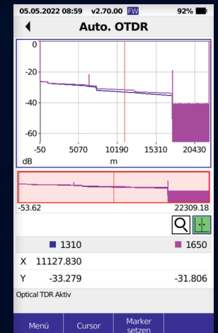
Grafik Auto-OTDR
