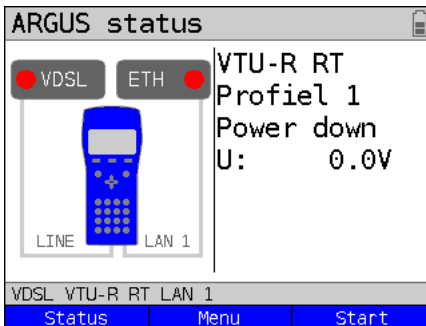
Afbeelding 2 (voorbeeld VTU-R-router):
